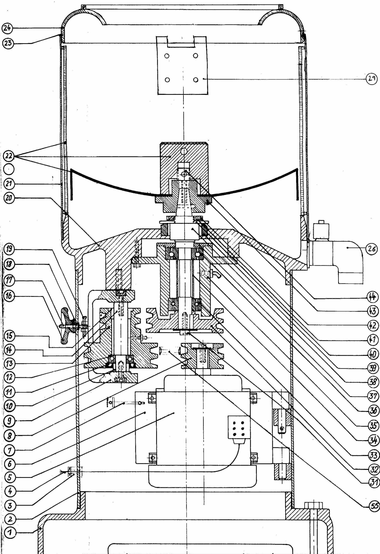
Aufbauzeichnung Schälmaschine 25 K VAP
