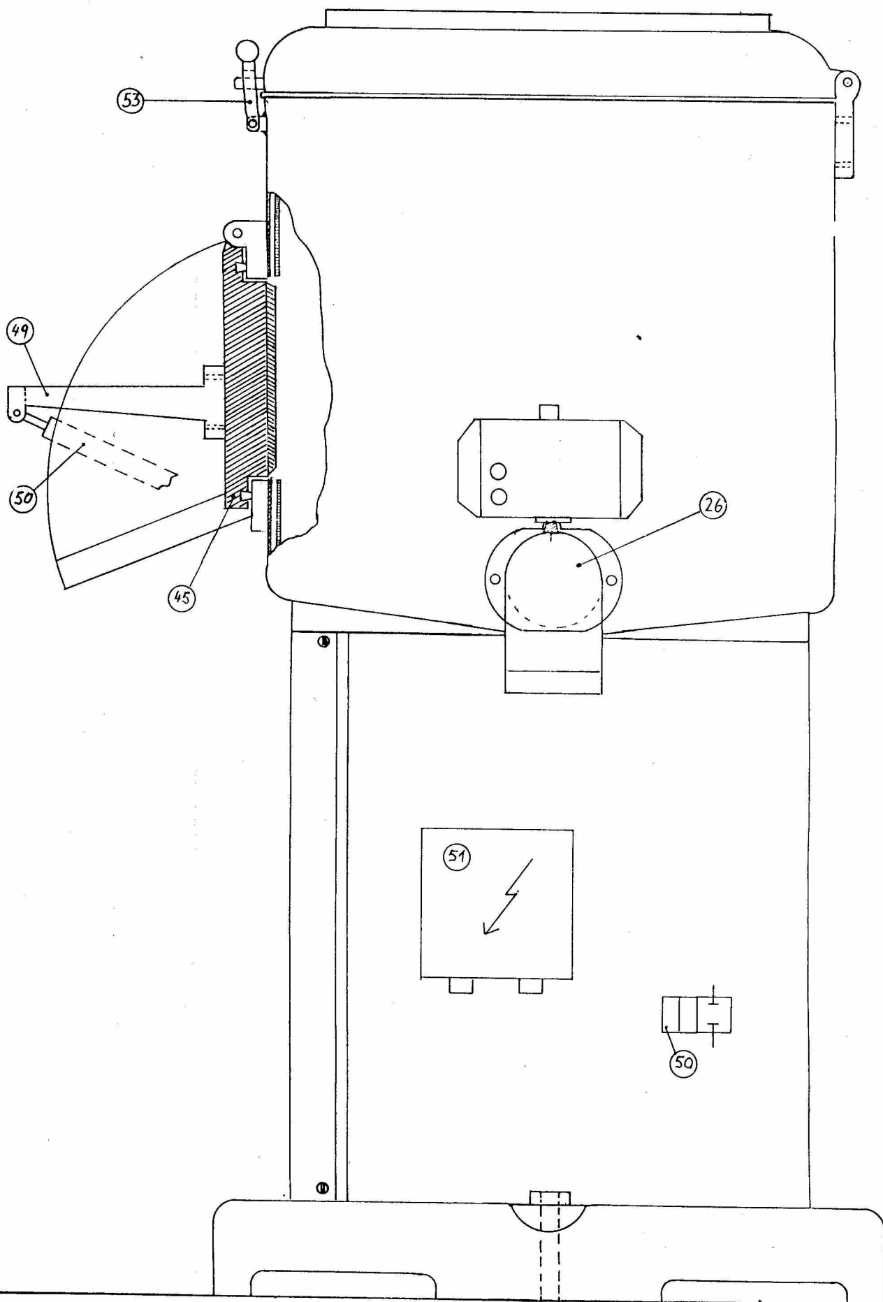
Aufbauzeichnung Schälmaschine 25 K VAP
